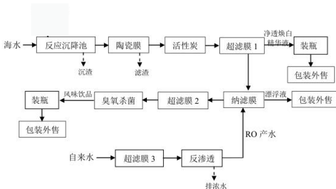
图 3.6-1 本项目生产工艺流程图
