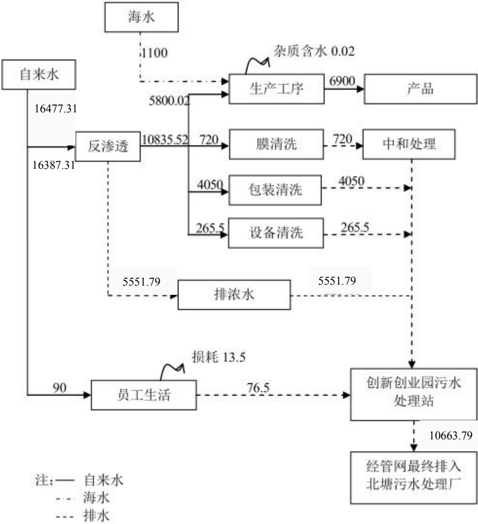
图 3.5-1 本项目水平衡图 (单位: \text{m}^3/\text{a} )
