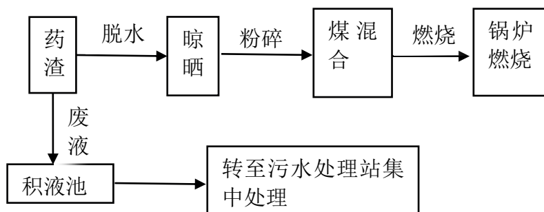
图 3-2 药渣处理工艺流程图（实际运营）
